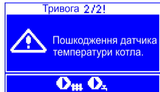
Мал. 29 Вигляд тривоги „пошкодження датчика температури котла”.
