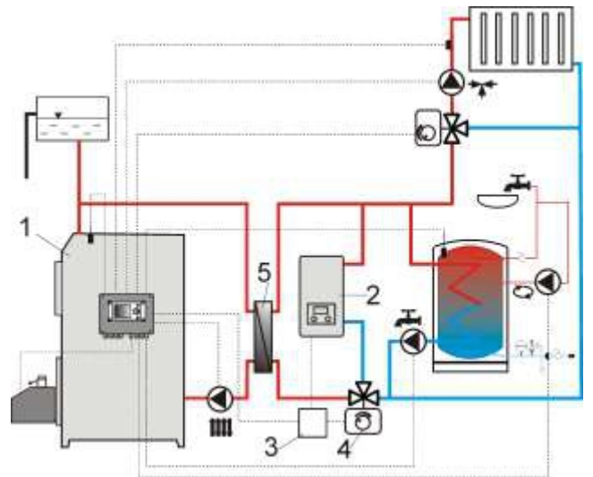
Рис. 25 липня Гідравлічна схема з додатковим котлом в відкритій - замкнутий контур, де : 1 - контролер, 2 -додатковий котел, 3 - передавач, 4 - перемикання клапан (з кінця комутатори), 5 - теплообмінник,
