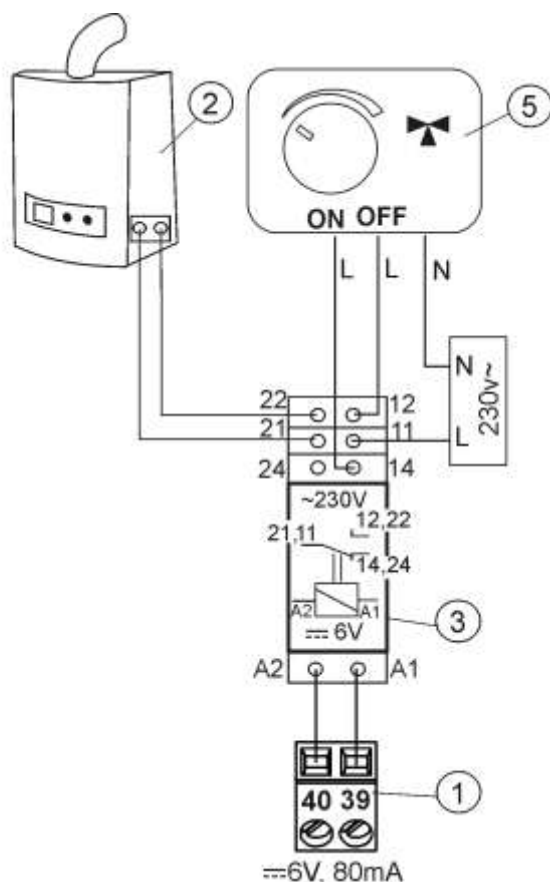
Мал. 26 Електричні схеми управління контактором додаткового котла, де: 1-контролер, 2-додатковий котел, 3-контактор, 5 - сервопривід клапана змішувача (з мікроками), увага: клеми 22, 21, 24 повинні бути відокремлені від клем 12, 11, 14.
