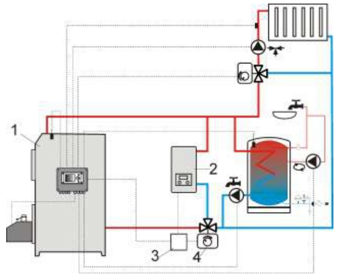
Мал. 24 6 Гідравлічна схема з додатковим котлом в замкнутій системі, де: 1-контролер, 2-додатковий котел, 3-контактор, 4-сервопривід клапана (з мікрореле).
