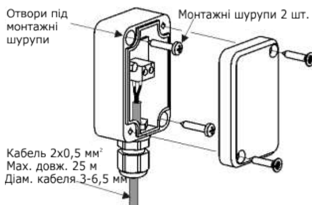
Мал. 23 Підключення зовнішнього датчика СТ4-Р.
