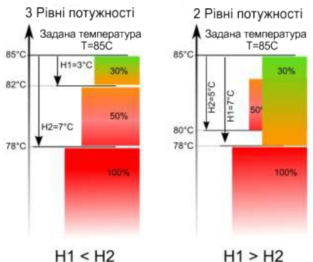
Мал. 8 Гістерезис H1 та H2 модуляції потужності.
